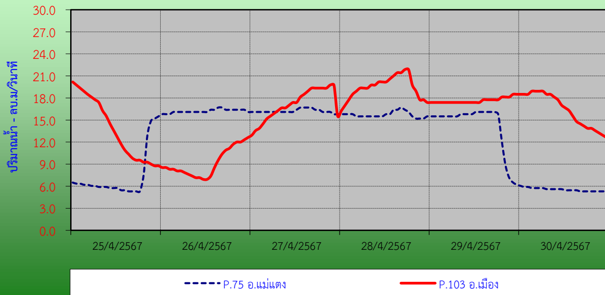
กราฟแสดงปริมาณน้ำปิ้งรายชั่วโมงรอบวันที่ 17/2567 ที่สถานีแม่ น้ำปิ้ง ( P.75) บ้านซ้อแล อ.แม่แตง และที่สถานีแม่ น้ำปิ้ง (P.103) บ้านป่าซ้อยใต้ อ.เมือง จ.เชียงใหม่
